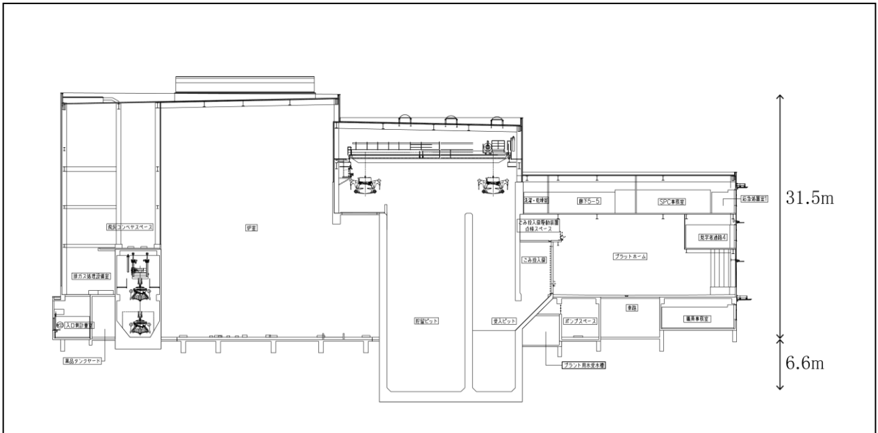
図1.5 断面図
