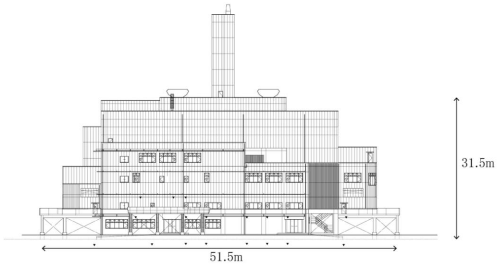
图1.6 立面图
