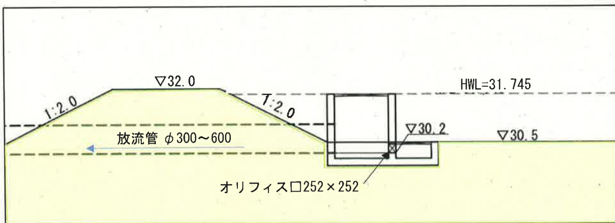
雨水流出抑制施設計画断面図（参考図）
