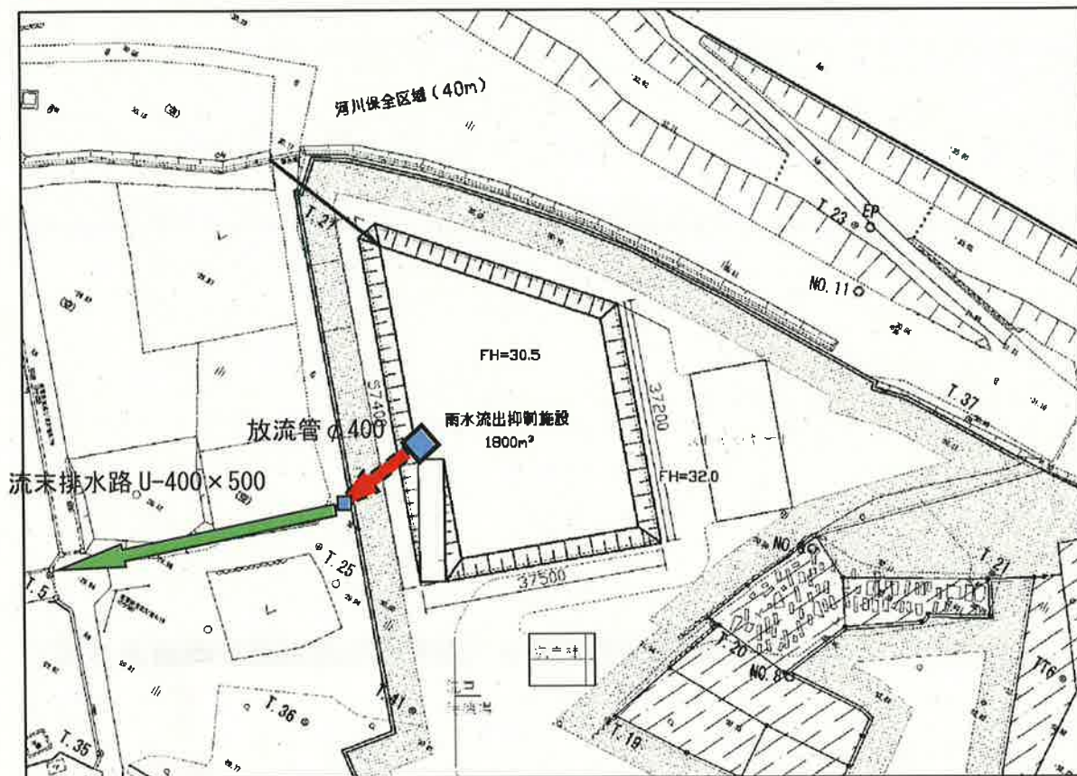
雨水流出抑制施設計画平面図（参考図）
