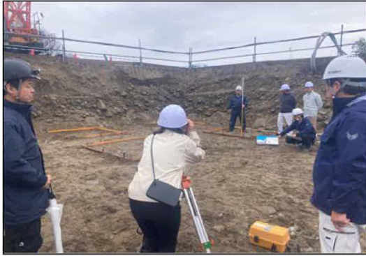
支持地盤確認
