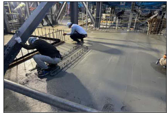
左官工事 コンクリート均し状況
